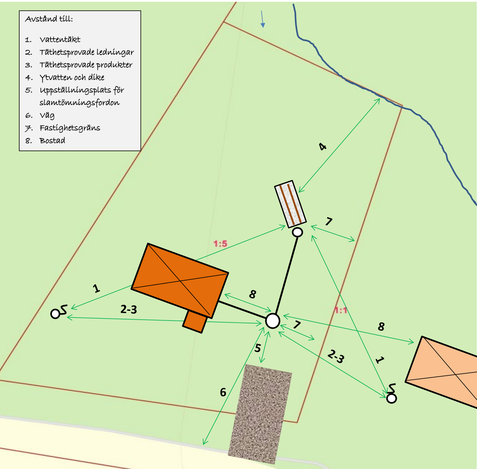
Figur 2. Horisontella skyddsavstånd
